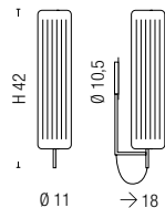
0037 1 x max 70W E27
