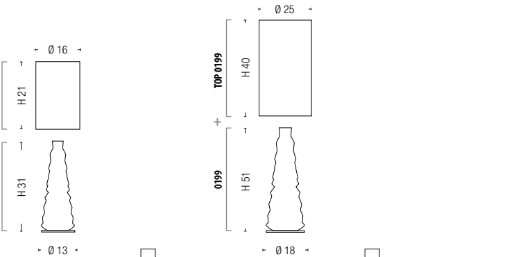
0198 + TOP 0198 = 1 x max 42W E14 0199 + TOP 0199 = 1 x max 70W E27
