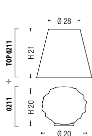
0211 + TOP 0211 = 1 x max 42W E14
