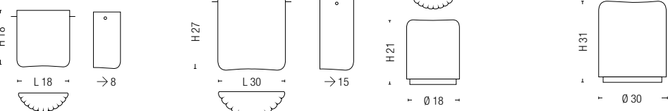
0126 1 x max 40W G9 0127 2 x max 42W E14 0128 1 x max 42W E14 0129 1 x max 70W E27
