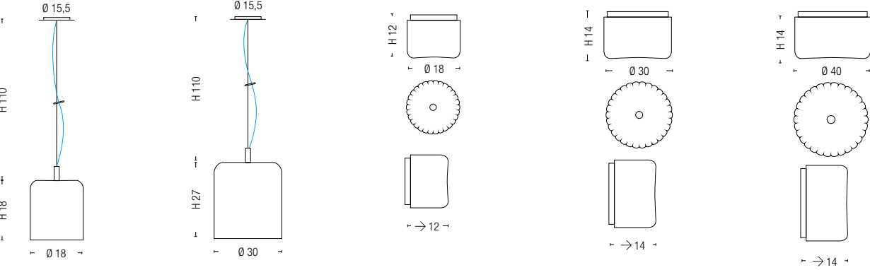
0122 1 x max 42W E14 0123 1 x max 70W E27 0120 2 x max 40W G9 0131 3 x max 42W E14 0121 4 x max 70W E27
