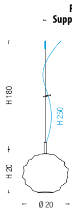
0202 1 x max 42W E14
