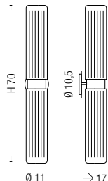
0039 2 x max 70W E27
