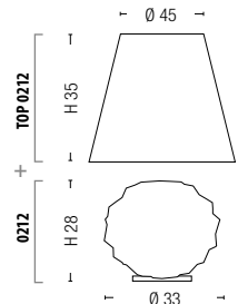
0212 + TOP 0212 = 1 x max 70W E27
