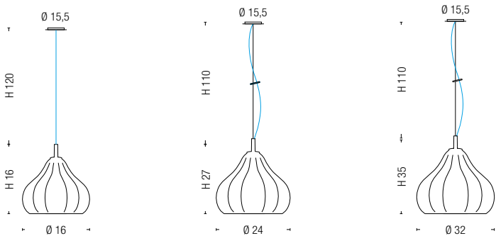
0240 1 x max 60W G9
