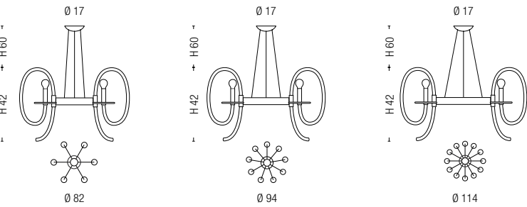
2050/6 6 x max 42W E14 2050/9 9 x max 42W E14 2050/12 12 x max 42W E14
