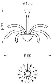
2030/15 CE 15 x max 25W G9
