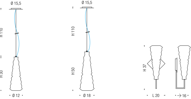
0190 1 x max 42W E14 0191 1 x max 70W E27 0194 1 x max 42W E14
