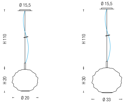
0200 1 x max 42W E14
