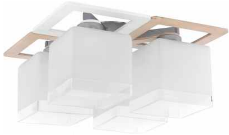
1454 XENA ceiling 18 cm 34 cm 34 cm 4 x E27, max 60W KL 7130
