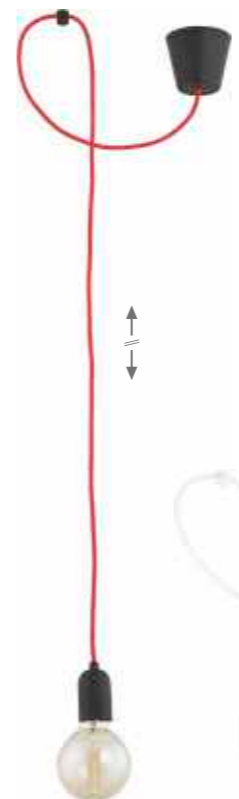
8631 QUALLE pendant lamp 170 cm 10 cm 10 cm 1 x E27, max 60W
