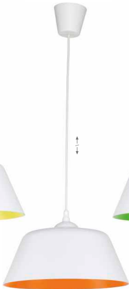
1703 ROSSI pendant lamp 90 cm 30 cm 30 cm 1 x E27, max 60W
